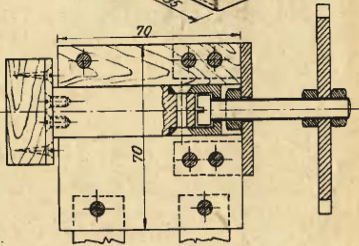
Csillagkerék 5. ábra.
