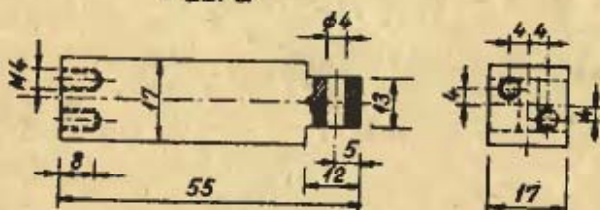
Tolórúd 1. ábra
