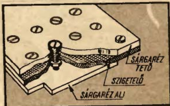
2. ábra. A nedvesség-érzékelő szerkezeti felépítése
