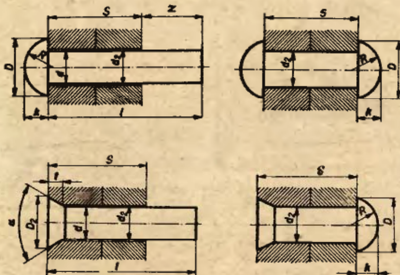
A lemezek közrefogása pl. félgömbfejú és süllyesztettfejú szegeccsel.
