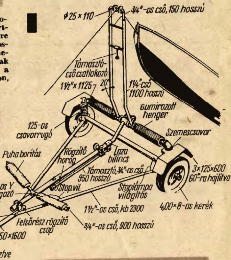
A csónakszállító kocsi elrendezése
