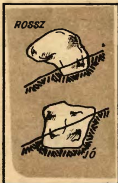
A szikla helytelen, illetve helyes beágyazása
