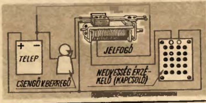
1. ábra. A jelzőberendezés áramköri kapcsolása
