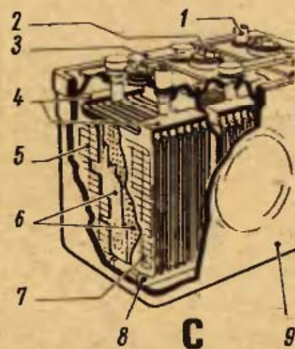
Az akkumulátor szerkezete; 1., negatív végkivezető, 2., menetes dugó, 3., összekötő sín, 4., pólushidak, 5., negatív lemezek, 6., elválasztó lemezek, 7., pozitív lemezek, 8., lemezeket tartó prizmák, 9., doboz
