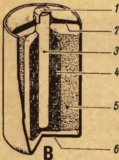
Egy szárazelem metszete; 1., fémfüveg, 2., szurokkiöntés, 3., szénpálca, 4., pozitív elektróda, 5., elektrolit, 6., horganytartály (anód)
