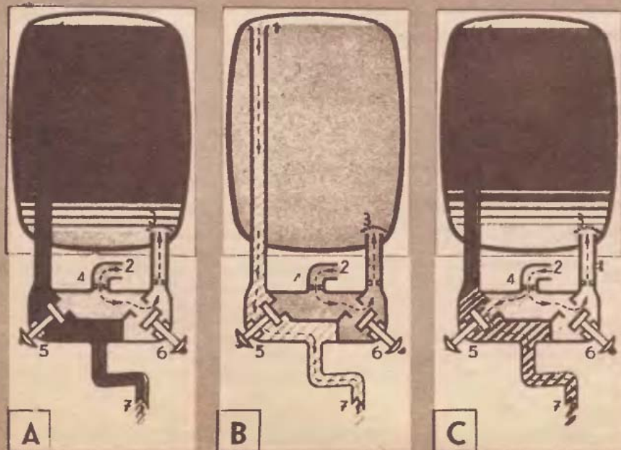
A kép — Megtöltés. B kép — Forró víz kivétel. C kép — Kevert víz kivétel. 1 — túlfolyócső, 2 — vízvezeték-csatlakozás, 3 — hideg víz beömlés, 4 — fojtó tárcsa, 5 — hideg víz szelep, 6 — forró víz szelep, 7 — lengő karos kiömlés
