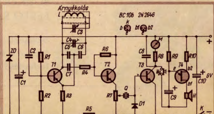
1. ábra. A „fémnyomozó” kapcsolási rajza. A készülék rejtett vezetékeit és fémtárgyakat műszerrel és hanggal egyaránt jelez
