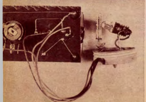
A szerelőlap huzalozása és a szabályozó elem csatlakozása
