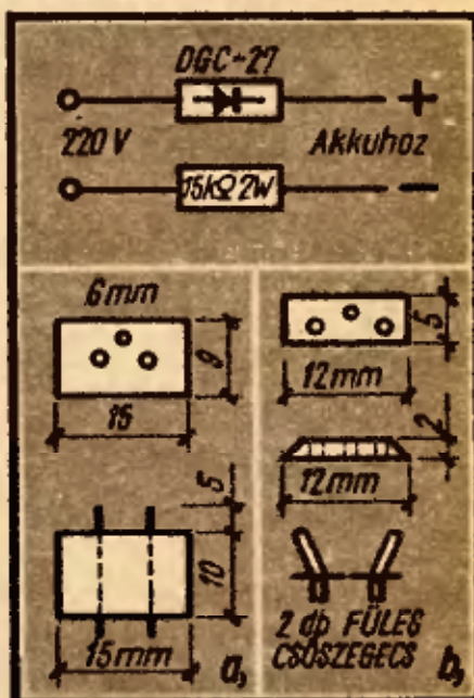
1. kép. Kulcslámpa, töltés közben
