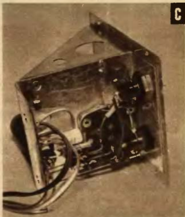
Címkép: Dobozba épített hőfokszabályozó és a forgatógombos hőérzékelő
