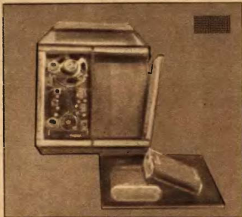
A másik kivitel két rétegeltlemez közé épített. Az egyik oldal kihajtható, az elemek cserélésekor a fedőlapot nem kell leszerelni
