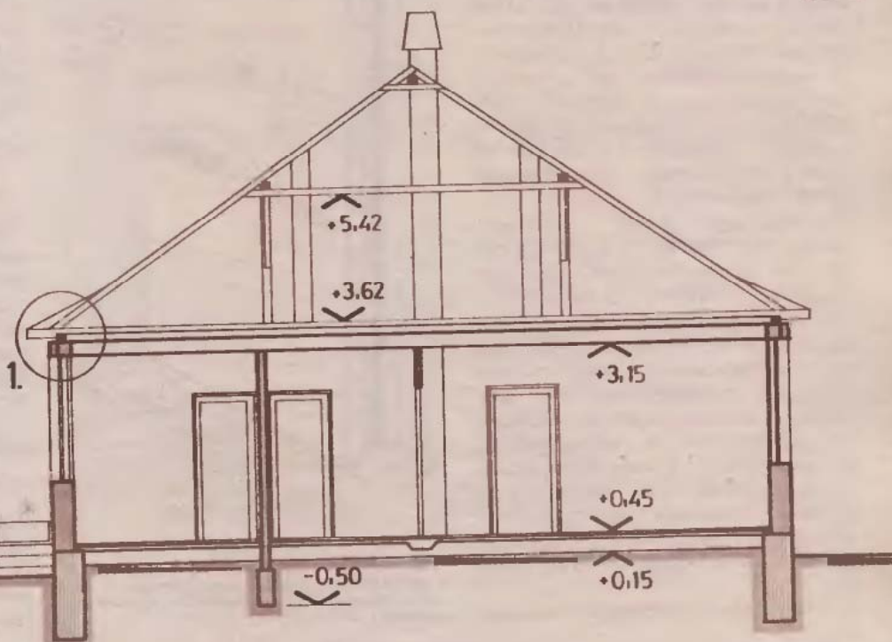
A-A METSZET
