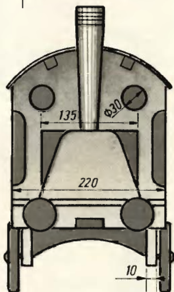
ELŐLNÉZET
