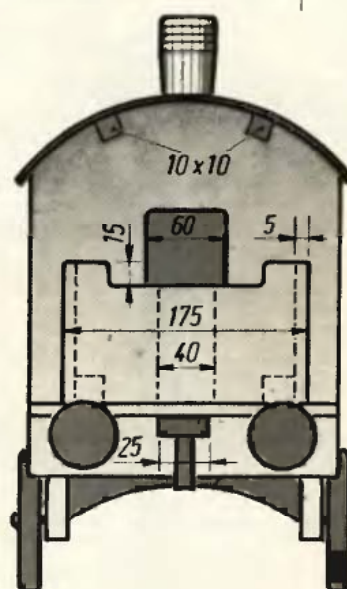
HÁTULNÉZET
