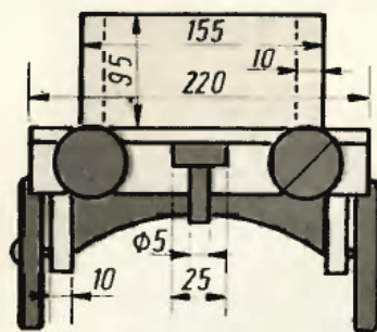
HÁTULNÉZET
