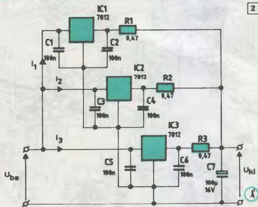
Három stabilizátor IC párhuzamos kapcsolása
