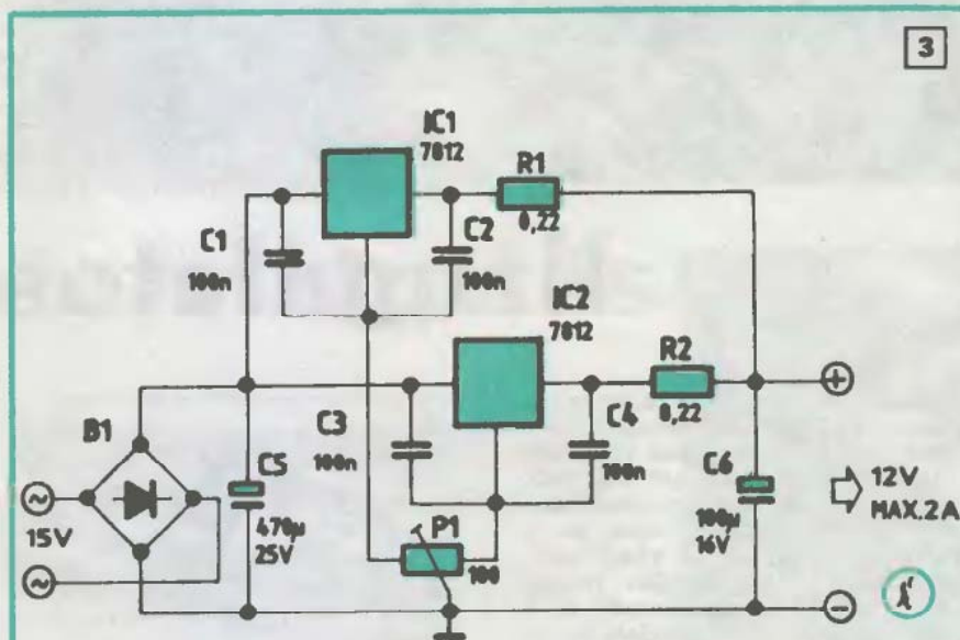
Két stabilizátor IC párhuzamos kapcsolása trimmerpotenciométeres kompenzációval
