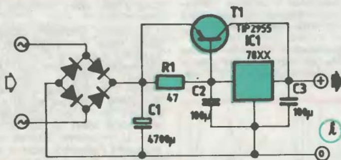
A kivehető áramerősség megnövelése teljesítménytranszisztor alkalmazásával
