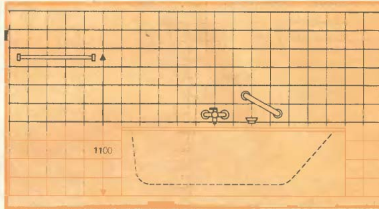
2. ábra. Itt a törülközőtartó, a szappantartó és a fogódzkodó kád körüli elhelyezése látható.
