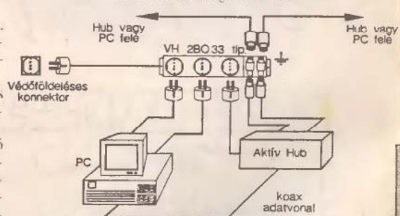
17. ábra Kapcsolási vázlat Arc Net hálózat (részlet) túlfeszültség-védelmére
