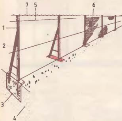
4. ábra Egyszerű áttört, védelmi funkciójú kerítés acéloszlopokkal, gépfonat kerítésmezővel
