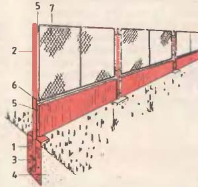
7. ábra Tömör lábazatú, acéloszlopos, keretre feszített acélhálós mezőjű kerítés
