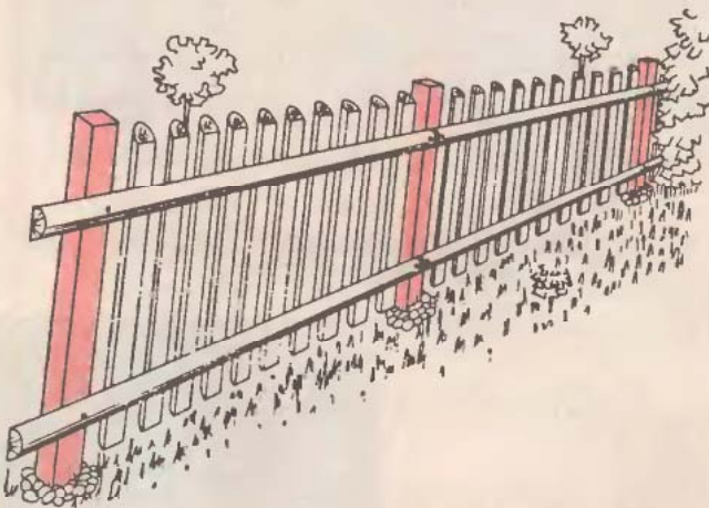
29. ábra Hosszirányban kettéfűrészelt gömbfa kerítés fűrészelt faoszlopokkal, félgömbfa hevederekkel
