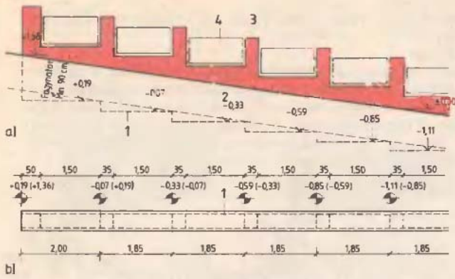
10. ábra Hagyományos kerítés lejtős terepen I.
