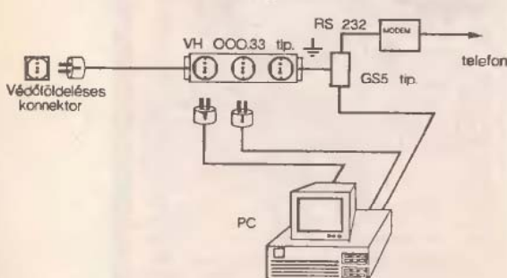
13. ábra Kapcsolási vázlat telefonvonalra kötött PC-k túlfeszültség-védelmére
