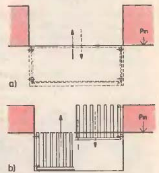
26. ábra. Emelkedő szárnyú kapuk
