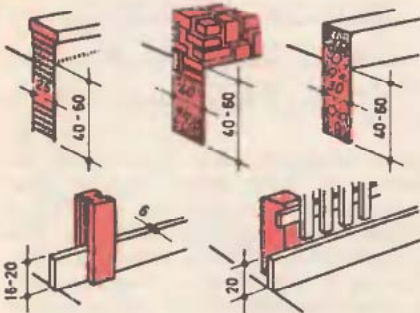
12. ábra Kerítésalapok és lábazatok
