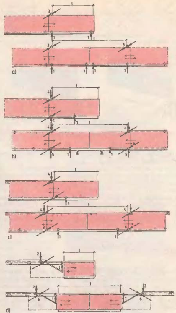
25. ábra Tolószárnyú kapuk működési elve
