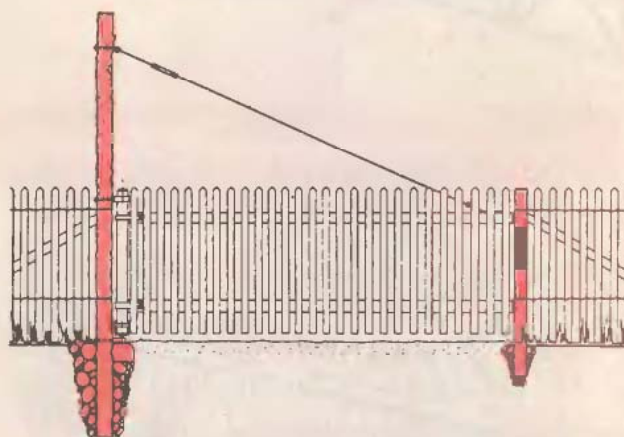
41. ábra Hagyományos buzalhevederes kerítés árboconra függesztett kapuval
