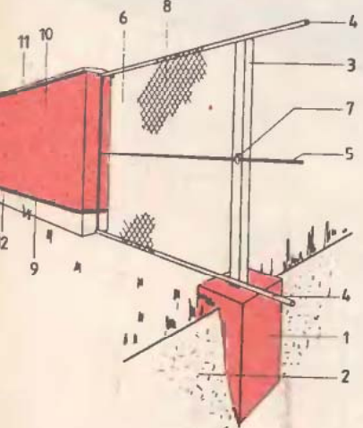
5. ábra Egyszerű áttört kerítés betonoszlopokkal, tömör mezőkkel
