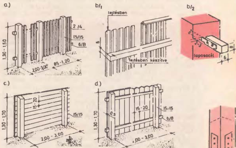
21. ábra. Fakerítések
