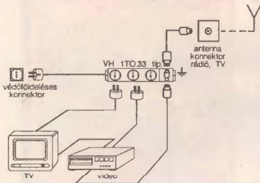
10. ábra Kapcsolási vázlat háztartási szórakoztató készülékek túlfeszültség-védelmére
