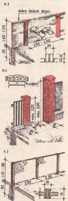
14. ábra Tégla-kerítés
