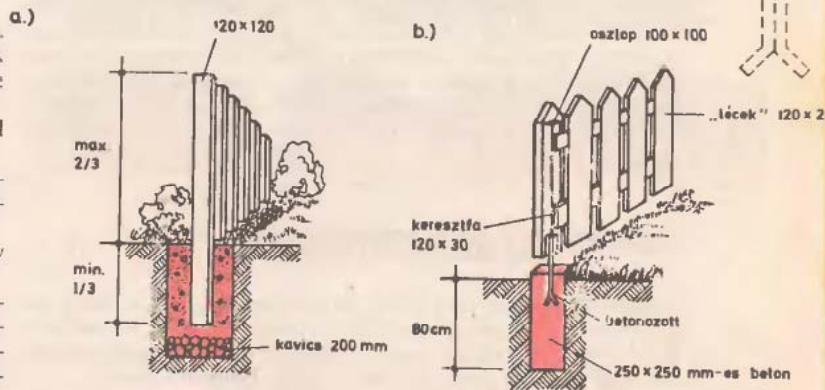
22. ábra. Fakerítések
