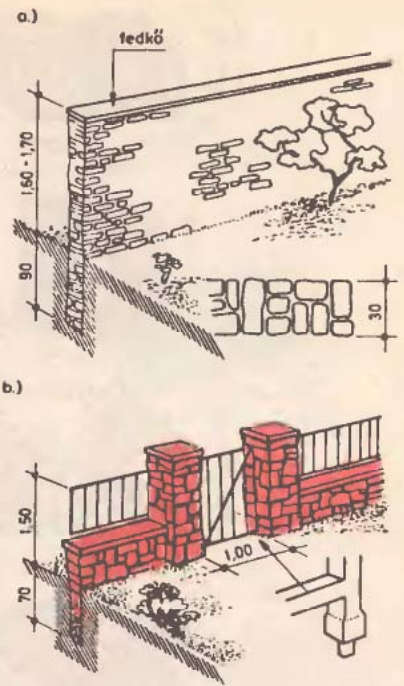
13. ábra Kőkerítések
