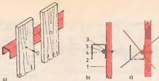
35. ábra Fémhevederes lécz, ill. deszkakerítések a – nézetrajz, b – helyes zárt, c – helytelen, felülről nyitott profilos megoldás, 1 – lécz vagy deszka kerítéselem, 2 – fémheveder, 3 – alátét, 4 – csavar, 5 – anyacsavar
