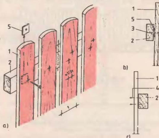
34. ábra Léckerítések korlátjainak, ill. hevedereinek kapcsolata
