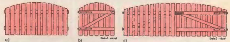
33. ábra Ívelt felső záródású léckerítés kerítésmezője, személy- és teherbejárati kapuja
