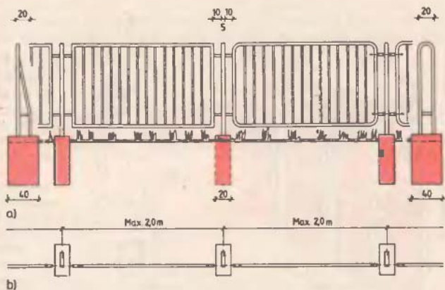
39. ábra Íves és szögletes kialakítású acélcső kerítés pontszerűen alapozott oszlopokkal a – nézet, b – alaprajz
