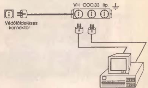
14. ábra Kapcsolási vázlat helyi számítógéprendszer túlfeszültség-védelmére
