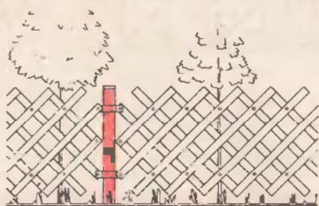
36. ábra Ferde lécezésű kerítéstípus faoszlopra szerelt változata
