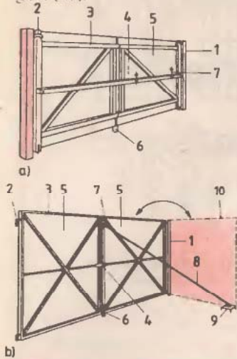
27. ábra Középen felnyíló kétszárnyú kapuk merevítése a – fakapu félmagasságban merevítőrúddal, b – acélkapu kitámasztórúddal, 1 – kapuoszlop, 2 – fordulópánt, 3 – keretheveder, 4 – zárheveder (merevítőrúd), 5 – kapuszárnyak borítása, 6 – ütköző zárretesszel, 7 – biztosítóhorog, 8 – támasztórúd, 9 – betontömbben elhelyezett horganyzószem, 10 – kapuszárny nyitott állapotban
