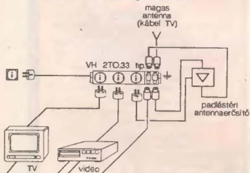
12. ábra Kapcsolási vázlat antennaerősítő túlfeszültség-védelmére
