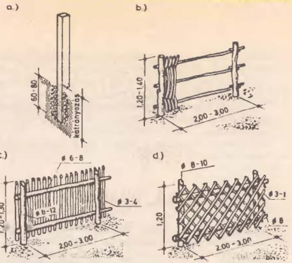
20. ábra. Fakerítések
