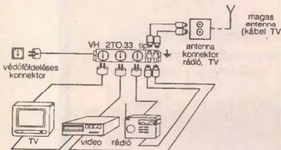
11. ábra Kapcsolási vázlat háztartási szórakoztató készülék túlfeszültség-védelmére
