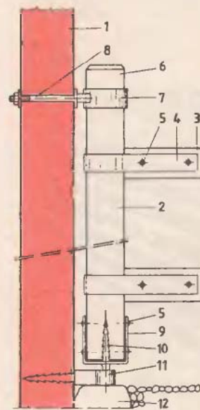
43. ábra Természetes alakú basított kővekből épített kerítésoszlop és lábazat lécezett fabetétel és kapukkal
