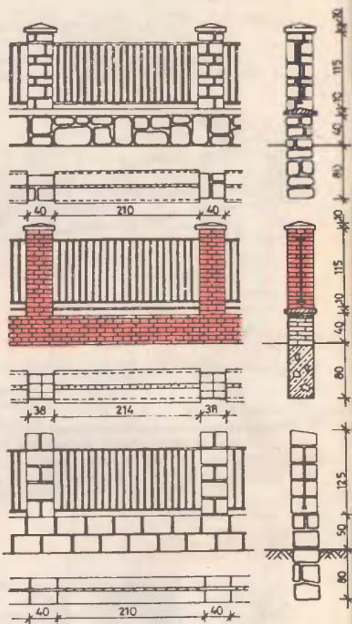
16. ábra Acélbetétes téglá- és kőkerítések
