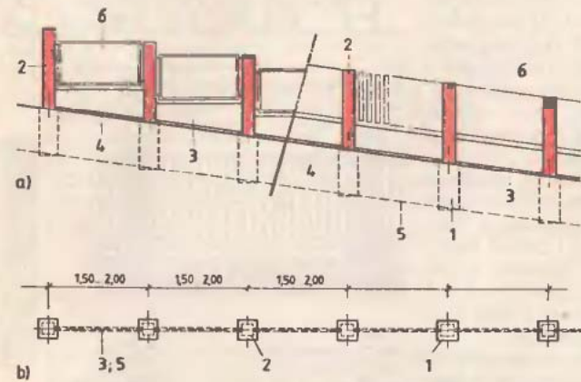
11. ábra Hagyományos emelt lábazatú kerítés lejtős terepen II, lépcsőzött és lejtővel párhuzamos kialakítás
