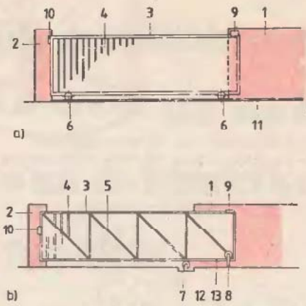
a – alsó gördülő megtámasztású, felső vezetési egyszárnyú tolókapu, b – konzolos tolókapu kombinált görgős felső vezetéssel, 1 – csatlakozó kerítésmezők, 2 – kerítésoszlop, 3 – kapuszárnykeret, 4 – kapuszárnyborítás, 5 – merevítő rácsolat, 6 – alsó görgő, 7 – támasztógörgő, 8 – lehorgonyzógörgő a konzolos működéshez, 9 – vezetógörgő, 10 – zárható ütköző, 11 – gördülőcsín, 12 – alsó és 13 – felső görgős kapuszárny
