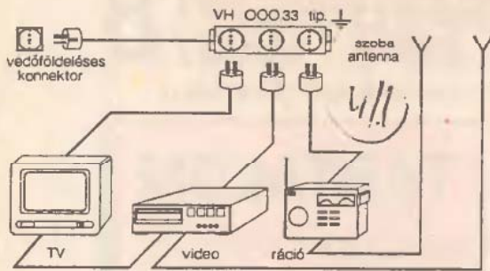
9. ábra Kapcsolási vázlat háztartási szórakoztató készülékek túlfeszültség-védelmére
