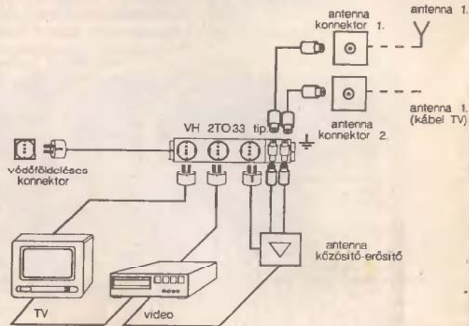
15. ábra Kapcsolási vázlat antennaerősítő túlfeszültség-védelmére
