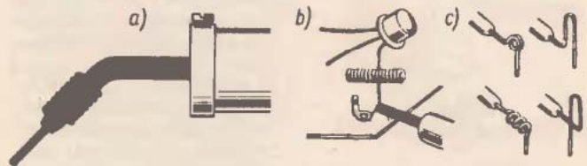
2. ábra A tranzisztoriábák forrasztása
