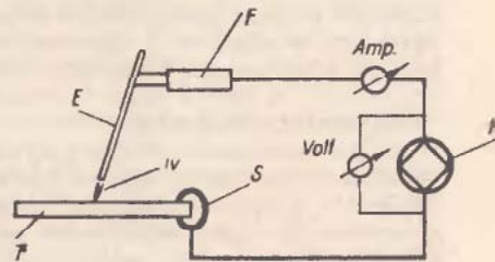
11. ábra Kézi ívhegesztés vázlatos elrendezése
