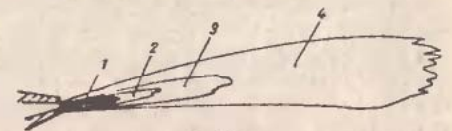
9. ábra A helyesen beszabályozott láng vázlat
