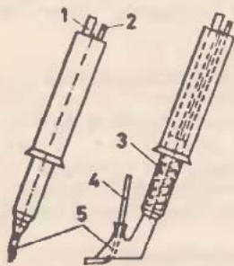
19. ábra Forrólevegős műanyaghegesztő készülék 1 – forró levegő beállítása, 2 – villamos csatlakozás, teljesítmény beállítása, 3 – cserélhető villamos fűtőtest, 4 – hegesztőpálca, 5 – hegesztőfúvóka
