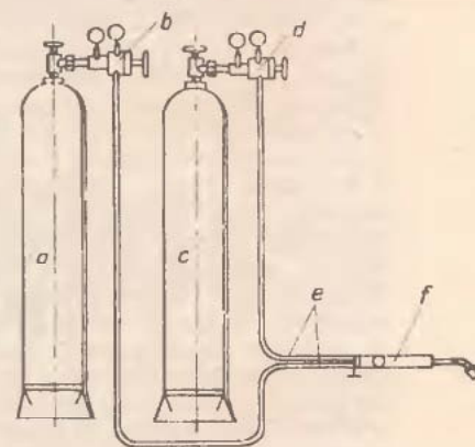
4. ábra Lánghegesztő-berendezés
