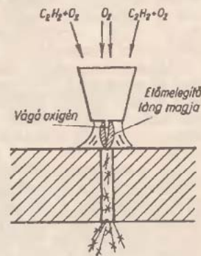
15. ábra Lángvágás sémája
