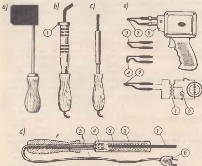
1. ábra Forrasztópákák
