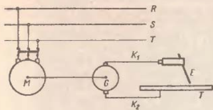
13. ábra Hegesztőgépcsoport elrendezési vázlat
