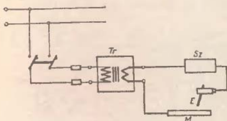
14. ábra Transzformátoros hegesztés sémája
