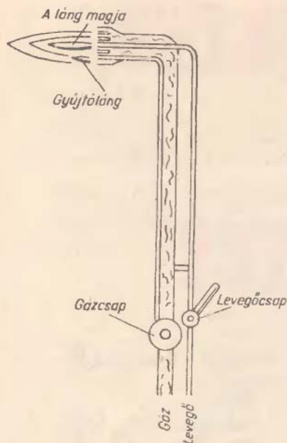
3. ábra Forrasztópisztoly
