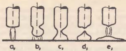
10. ábra Cseppképződés és anyagátvitel ívhegesztésnél
